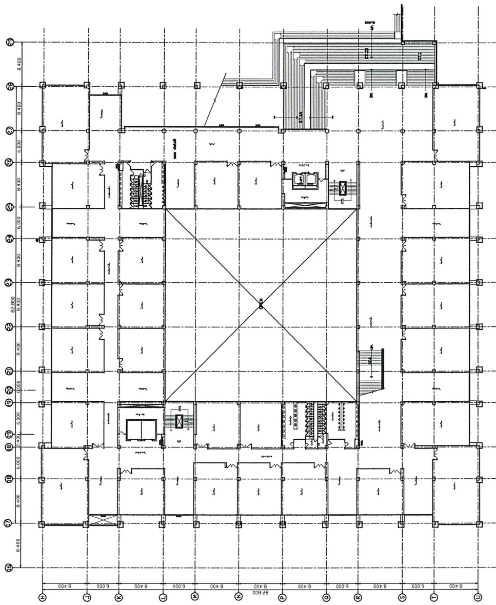
แปลนพื้นชั้น 2 SCALE 1:300
